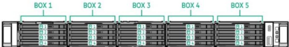
20 E3.S drive bay, SFF/EDSFF CTO server (P81966-B21)
